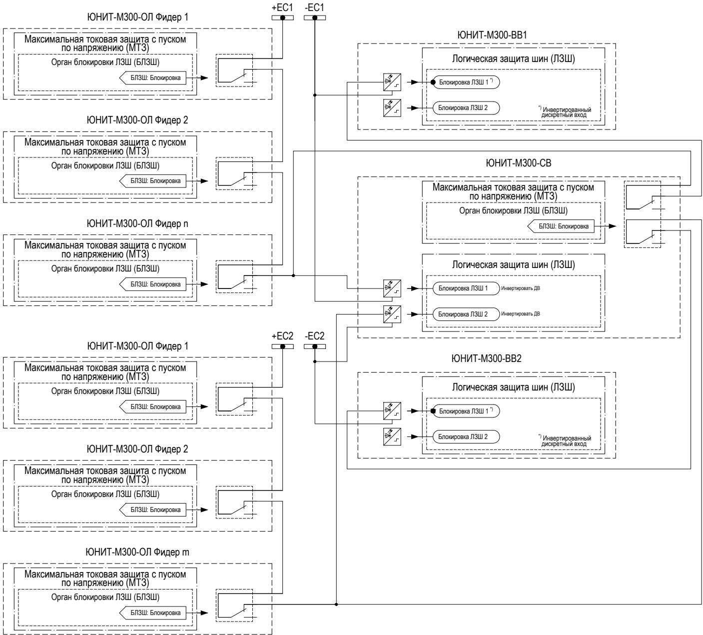
Рисунок Ж.2 – Последовательная схема организации работы ЛЗШ
