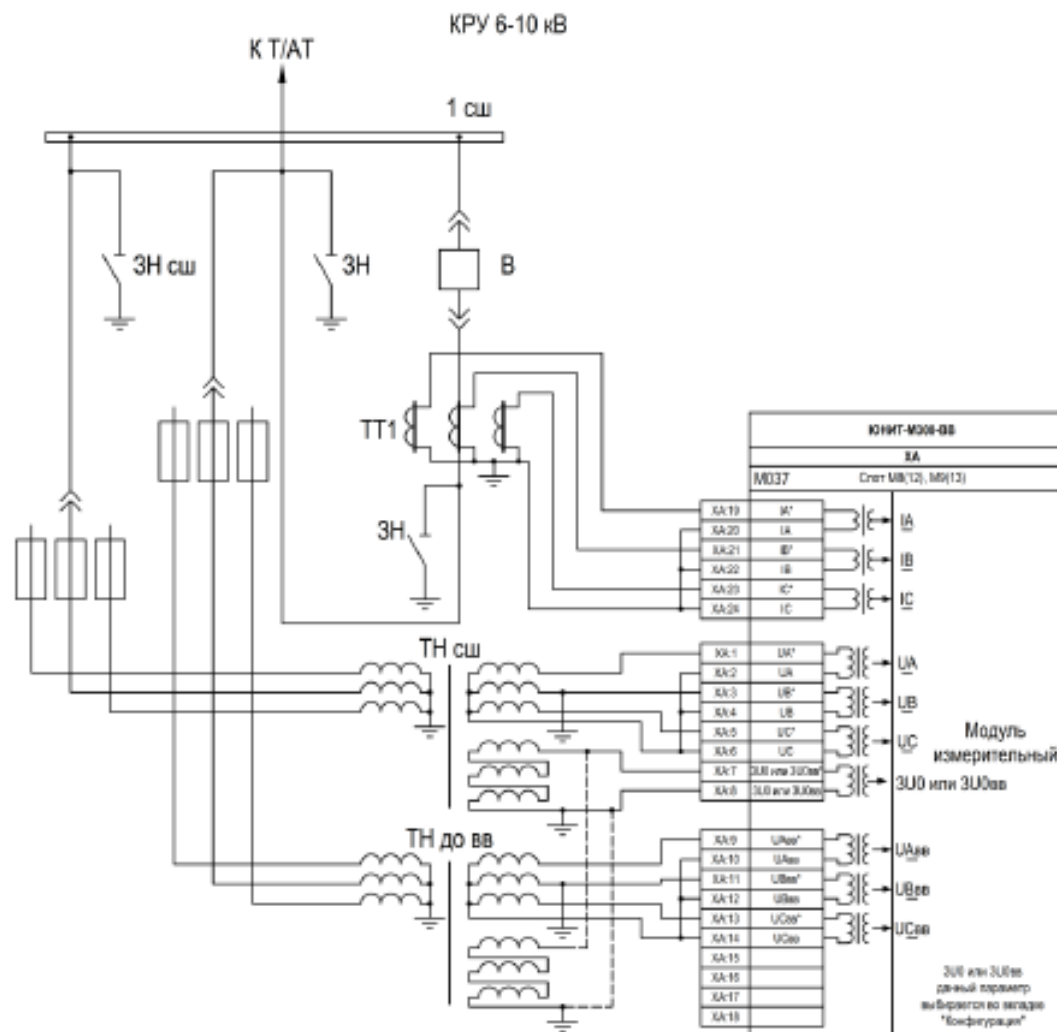
Рисунок В.1 – Пример подключения аналоговых цепей трансформаторов тока и напряжения
